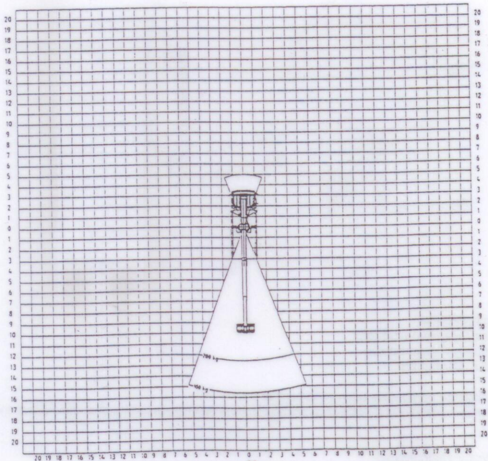
0° Kennfeld TKA 30 KS schmale Abstützung Fahrzeugbedingte Änderungen vorbehalten
