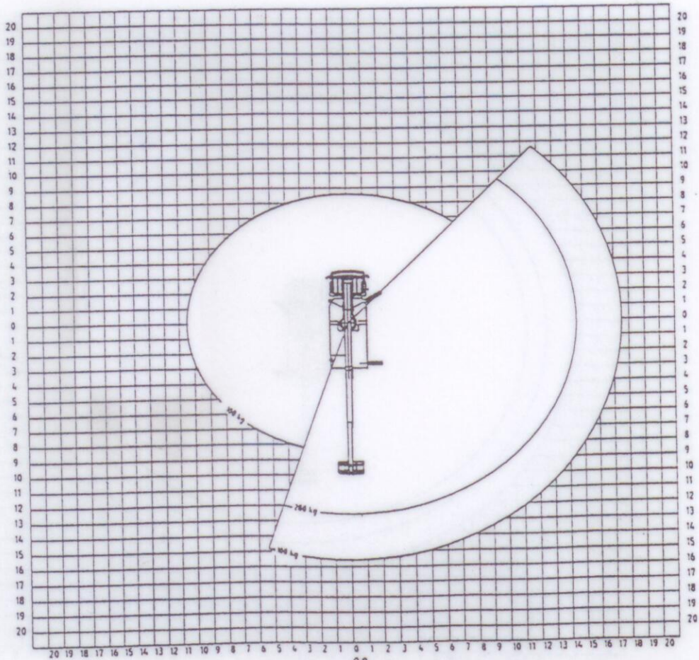
0° Kennfeld TKA 30 KS einseitige Abstützung Fahrzeugbedingte Änderungen vorbehalten
