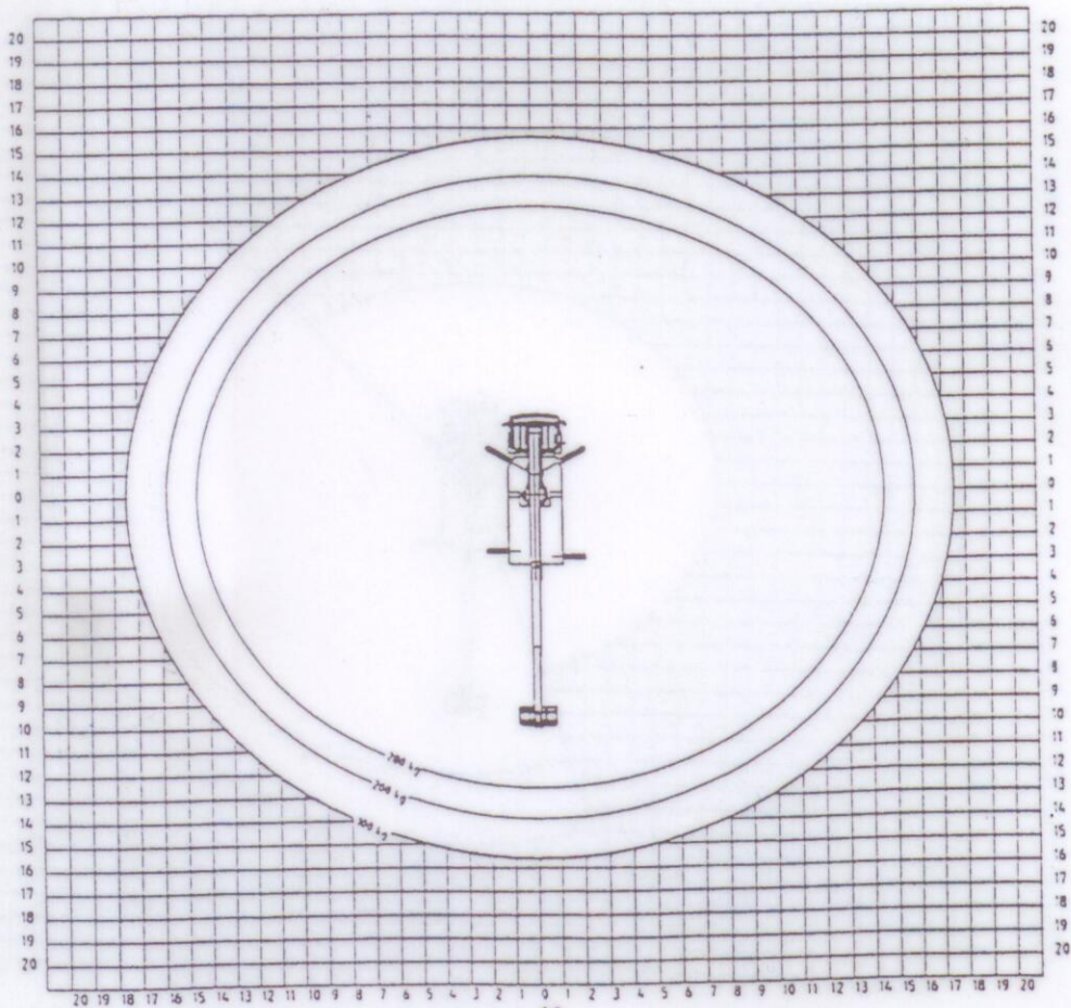
0° Kennfeld TKA 30 KS breite Abstützung Fahrzeugbedingte Änderungen vorbehalten
